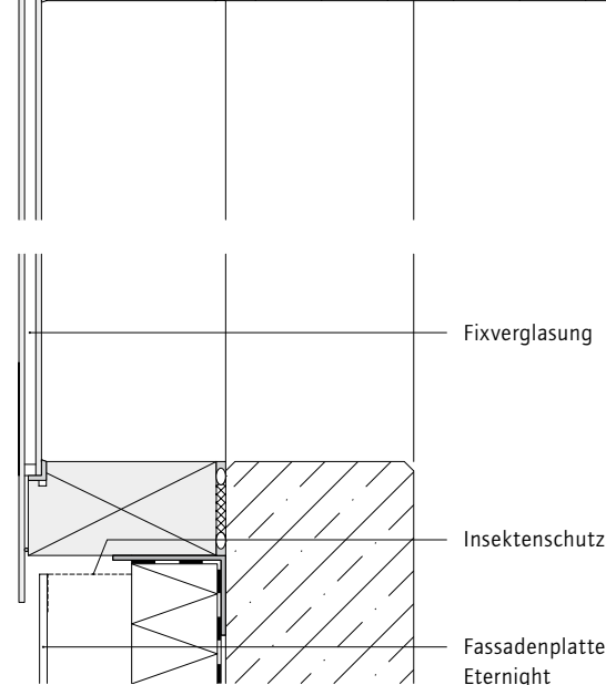
Fassadenschnitt
