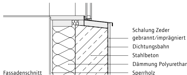
Fassadenschnitt
