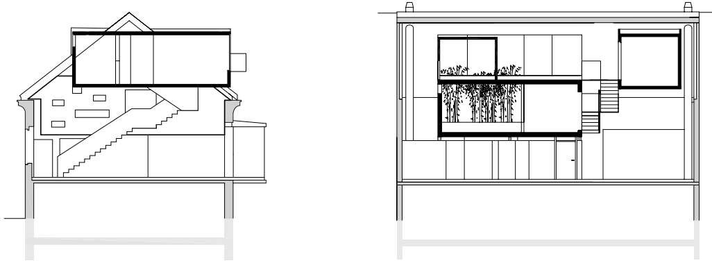
Quer- und Längsschnitt
