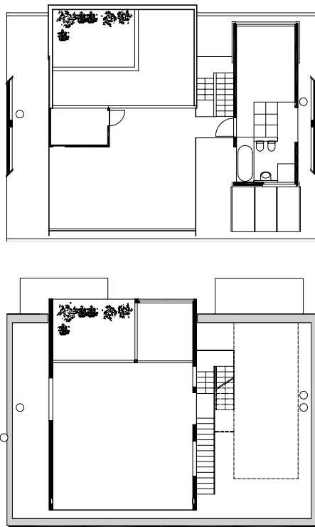
Grundriss obere und mittlere Ebene
