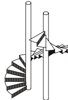
teilmgewundene Treppen symmetrisch mit einem geraden Antrittsarm und zwei gewundenen Austrittsarmen
