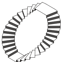
gewundene Treppen und Spiraltreppen symmetrisch mit zwei gewundenen Läufen
