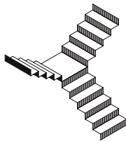
zweiläufig divergierend mit gemeinsamem Antritt und Zwischenpodest
