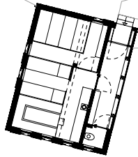
Grundriss Erdgeschoss Winterhaus und Hauptgebäude
